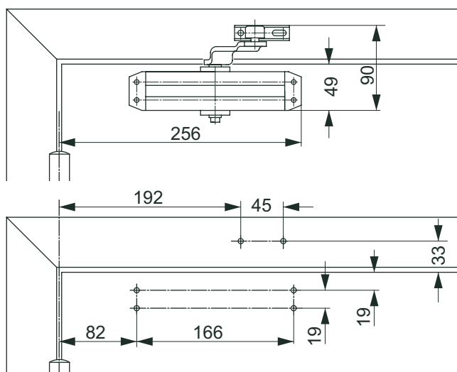
Montage sur la porte Le schéma montre l'application pour une porte gauche.
